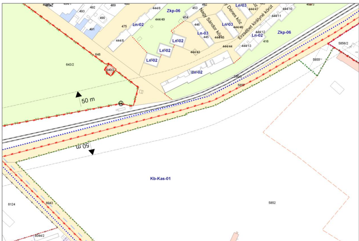
A Szabályozási Terv módosításának tervezete (részlet-2 | nincs változás)
