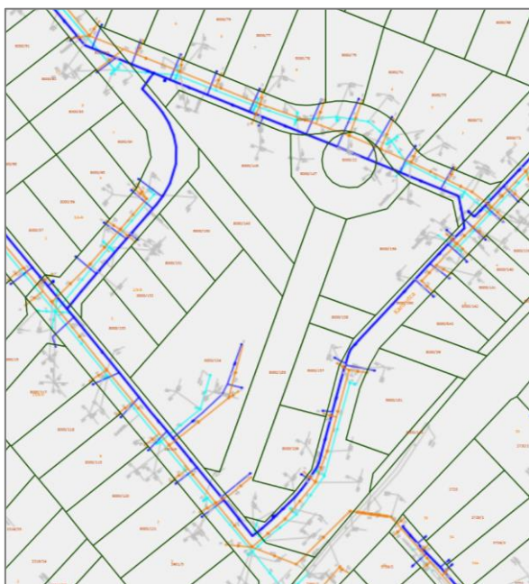
Víziközművek (forrás: önkormányzat)
