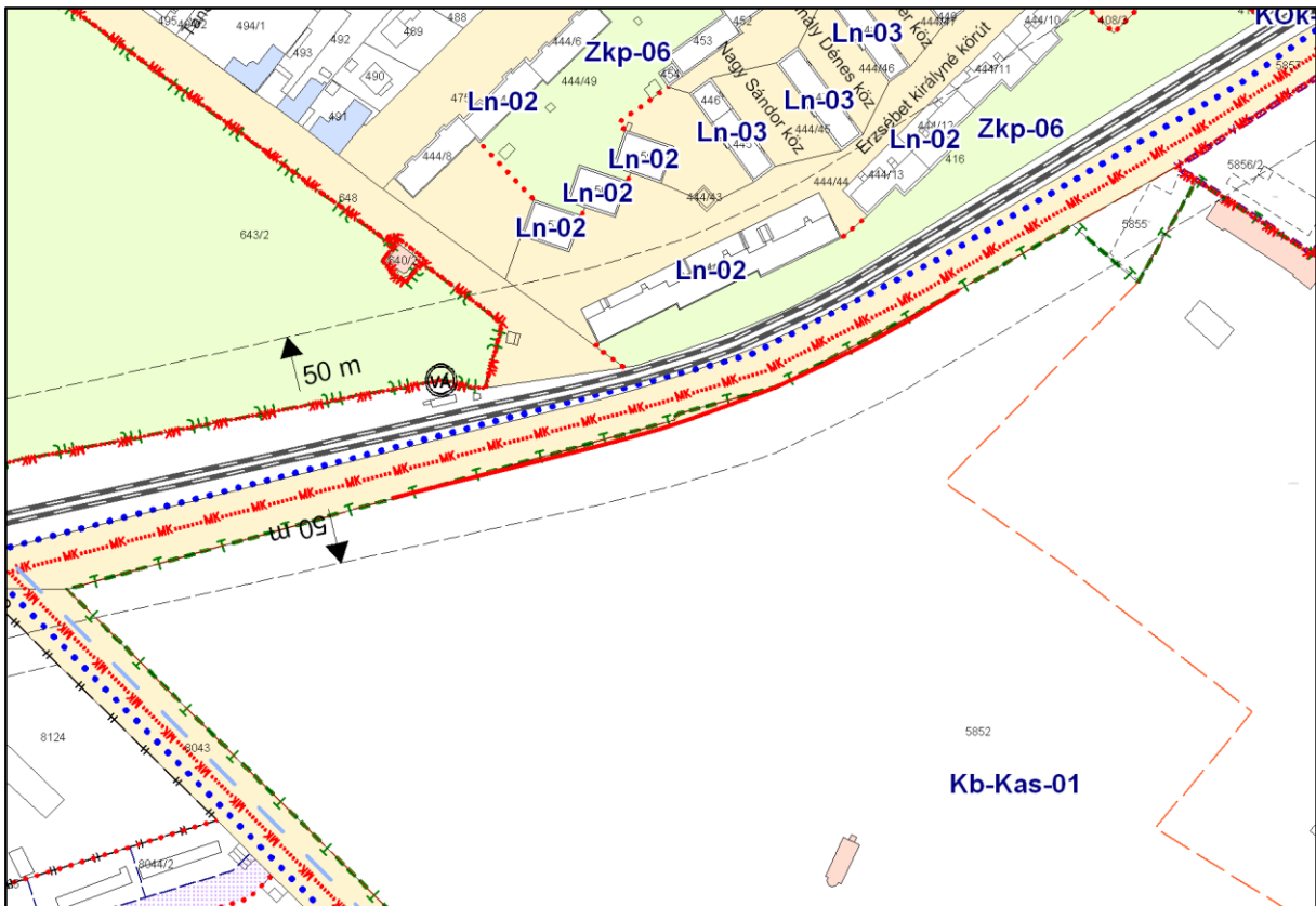
A Szabályozási Terv módosítása (Szabadság út)
