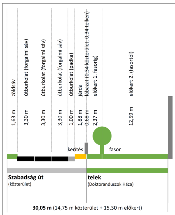
A Szabadság út meglévő keresztmetszete
