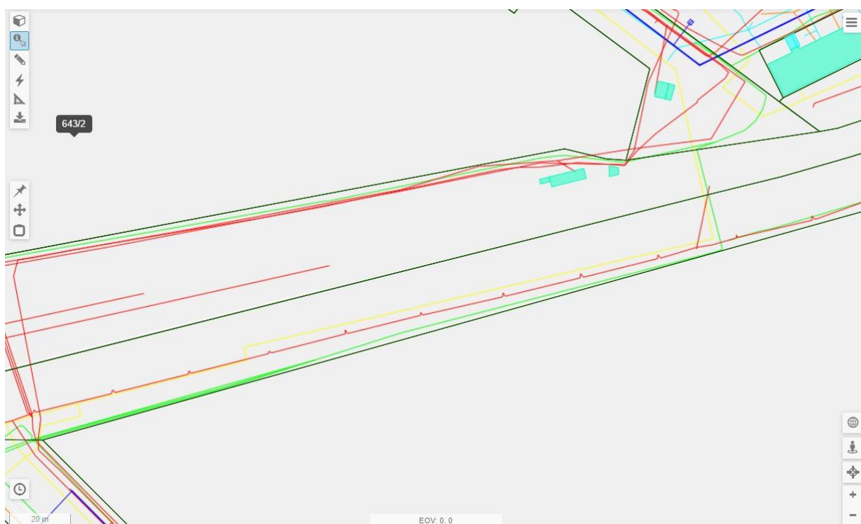
A Szabadság út érintett szakaszainak burkolatai és a közművek (forrás: Önkormányzat)
