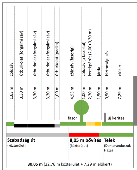
A Szabadság út tervezett keresztmetszete
