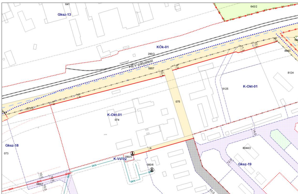
A Szabályozási Terv módosításának tervezete (részlet)
