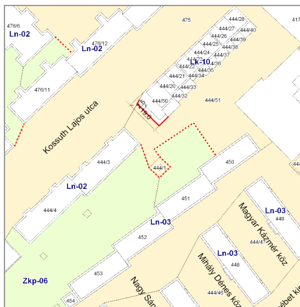
A Szabályozási Terv módosításának tervezete
